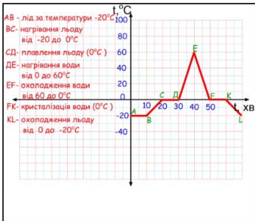
Рис. М.4. Smart-урок «Плавлення і кристалізація», графіки
