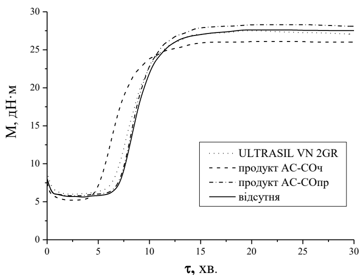
Рис. 2. Кінетичні криві сірчаної вулканізації (T=155°C) протекторних еластомерних композицій з різними типами мінеральних складових
