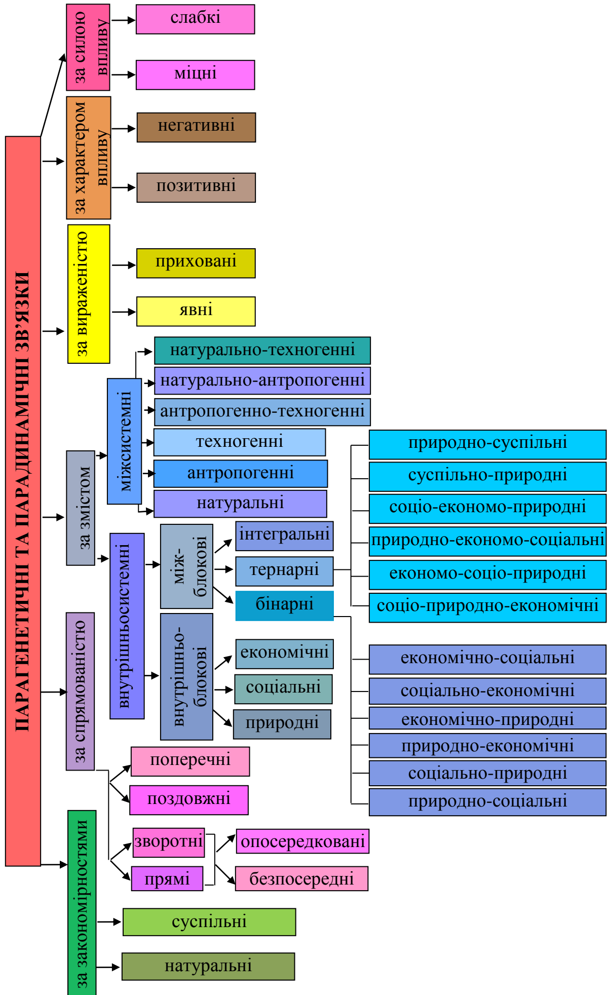
Рис. 3. Класифікація парадинамічних та парадинамічних зв'язків у ландшафтних системах
